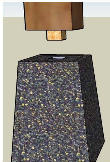
Gambar 6. Sistem kolom dan umpak
