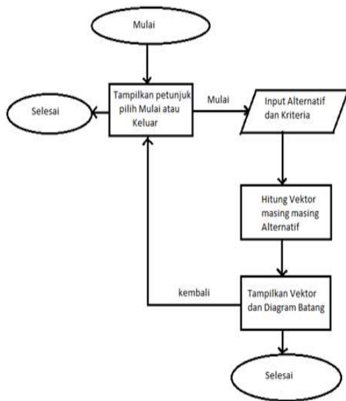
Gambar 5. Flowchart sistem aplikasi Pemanding Gitar
